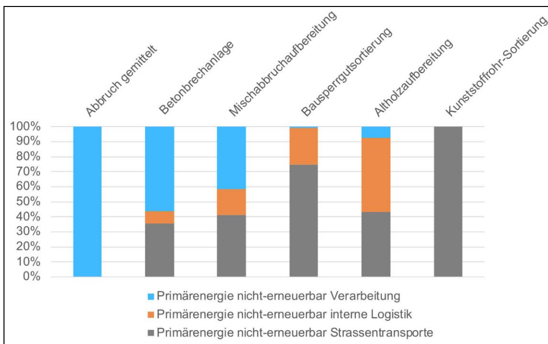
Abbildung 29: Anteile der Teilprozesse Transporte, interne Logistik und Verarbeitung an der aufgewendeten nicht-erneuerbaren Primärenergie der Entsorgungsprozesse
