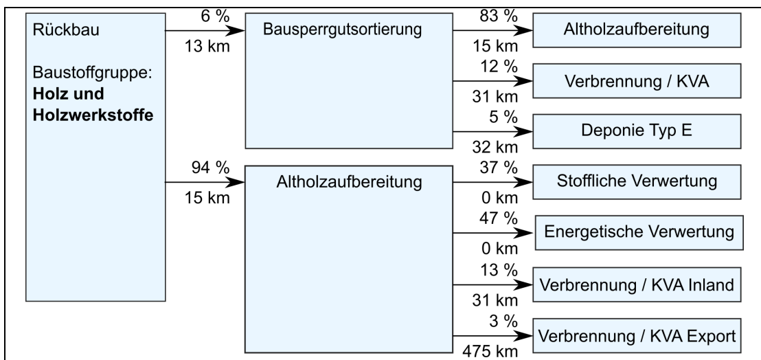
Abbildung 48: Entsorgungsweg Holz und Holzwerkstoffe
