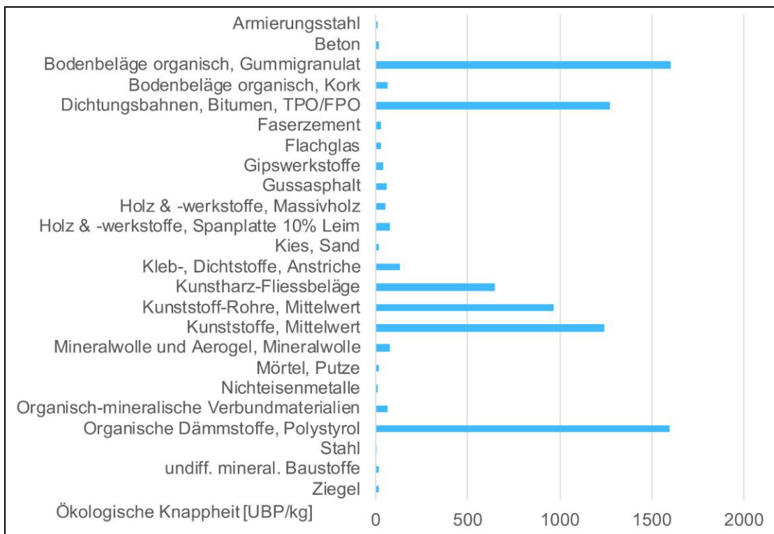
Abbildung 32: Ökobilanzergebnisse aller Prozessketten für die Umweltbelastungspunkte
