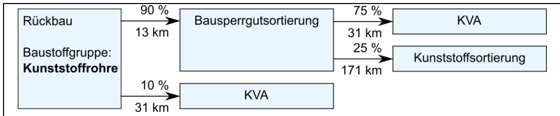
Abbildung 53: Entsorgungsweg Kunststoff-Rohre
