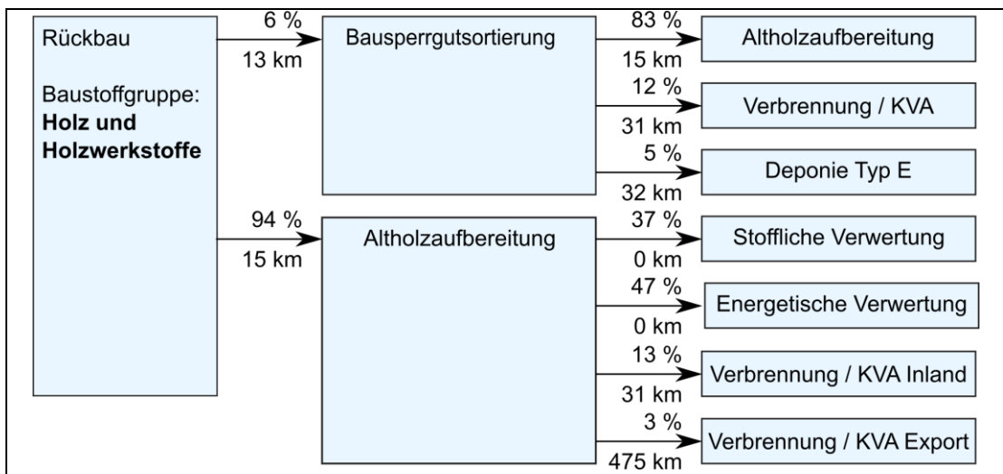
Abbildung 12: Entsorgungsweg Holz und Holzwerkstoffe
