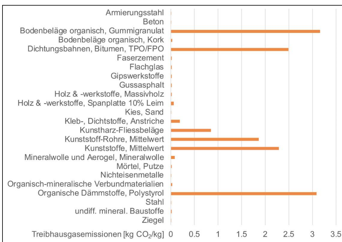
Abbildung 30: Ökobilanzergebnisse aller Prozessketten für die Treibhausgasemissionen
