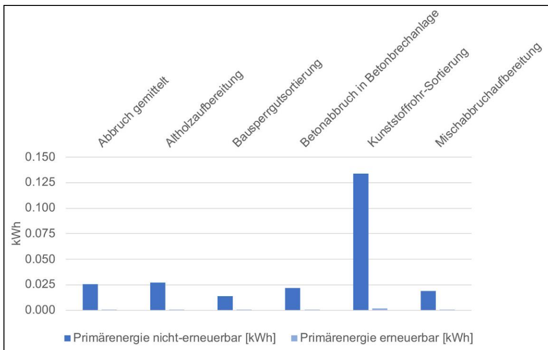
Abbildung 26: Ökobilanzergebnisse der Entsorgungsprozesse für Primärenergie pro Kilogramm Abfall
