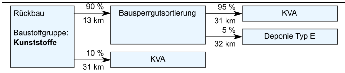
Abbildung 52: Entsorgungsweg Kunststoffe
