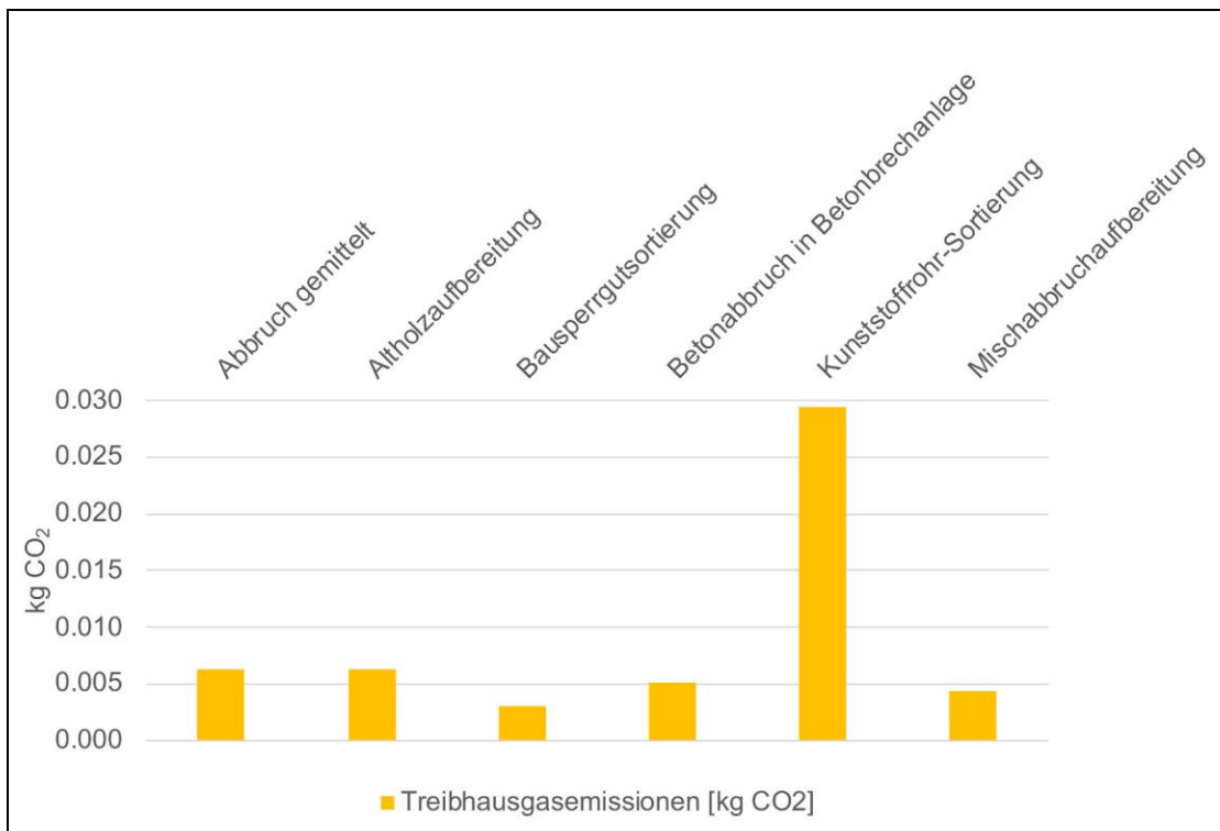
Abbildung 27: Ökobilanzergebnisse der Entsorgungsprozesse für Treibhausgase pro Kilogramm Abfall
