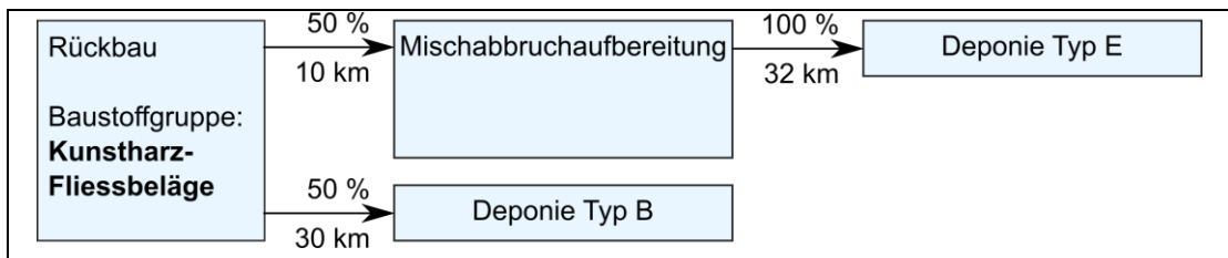
Abbildung 15: Entsorgungsweg Kunstharz-Fliessbeläge
