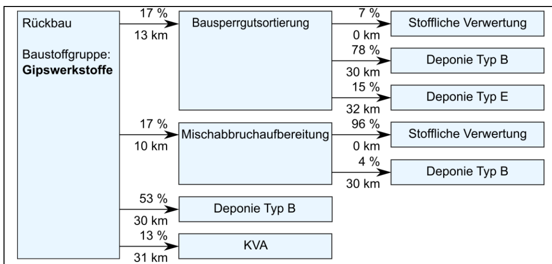
Abbildung 10: Entsorgungsweg von Gipswerkstoffen
