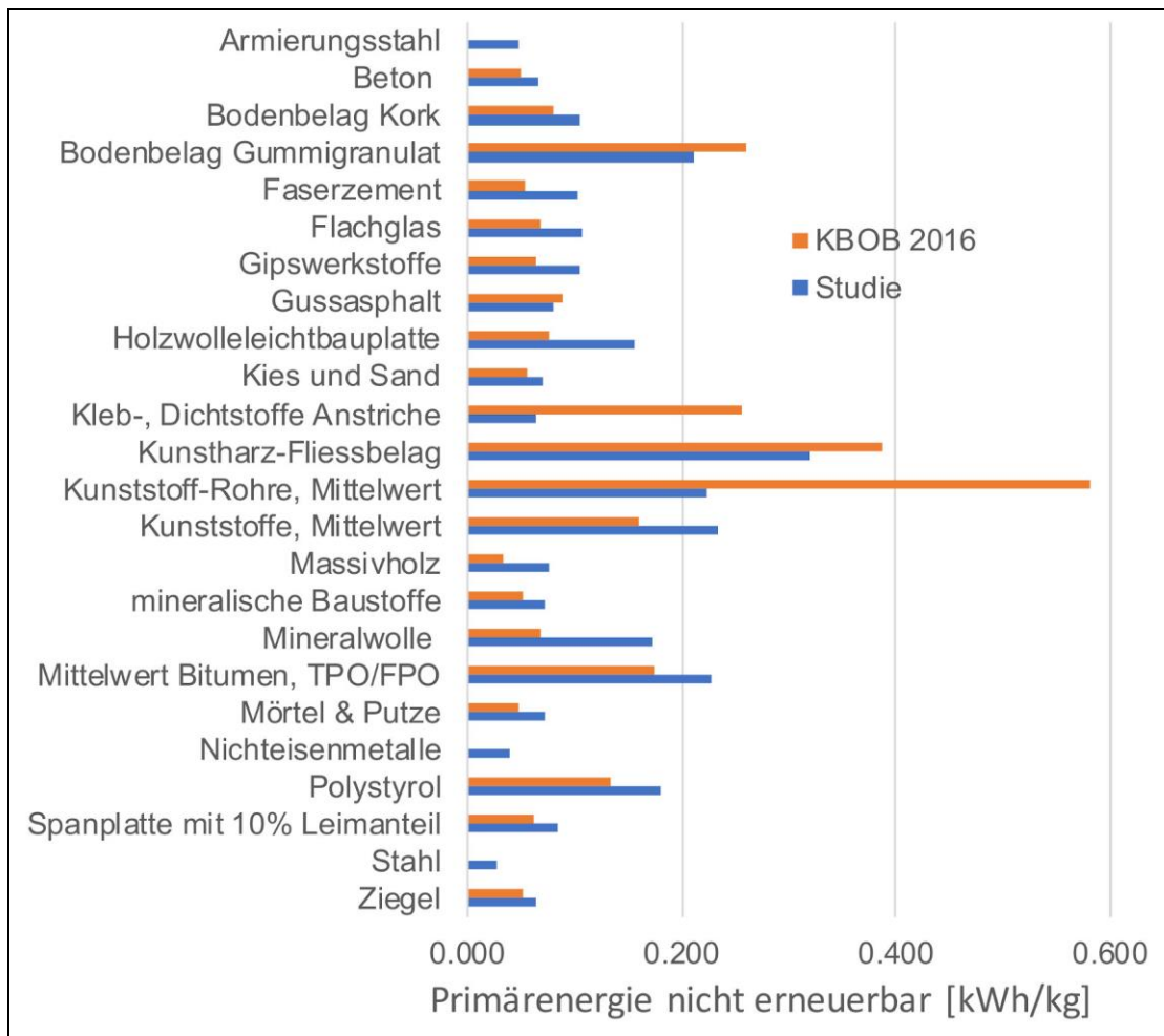
Abbildung 37: Vergleich mit KBOB-Daten, Primärenergie nicht erneuerbar
