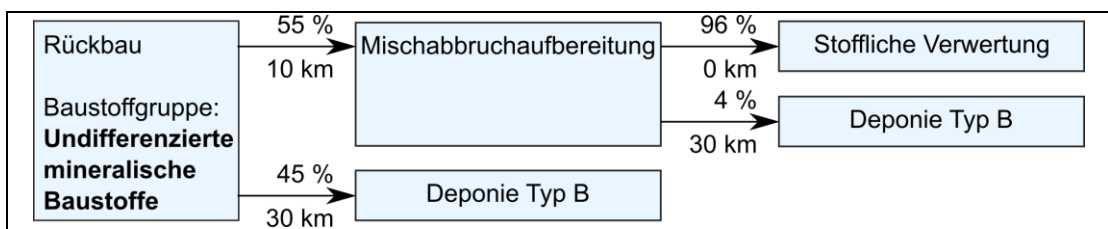
Abbildung 60: Entsorgungswege für undifferenzierte mineralische Baustoffe
